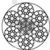
6×19S + IWR
