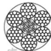
6×19W + IWR
