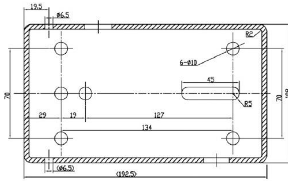
GJP400/WJP400安装尺寸
